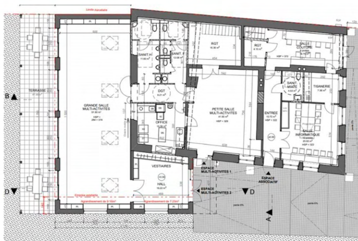
Plan de réhabilitation de la maison des associations
